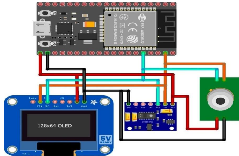
Gambar 3. Wiring Diagram Perancangan
