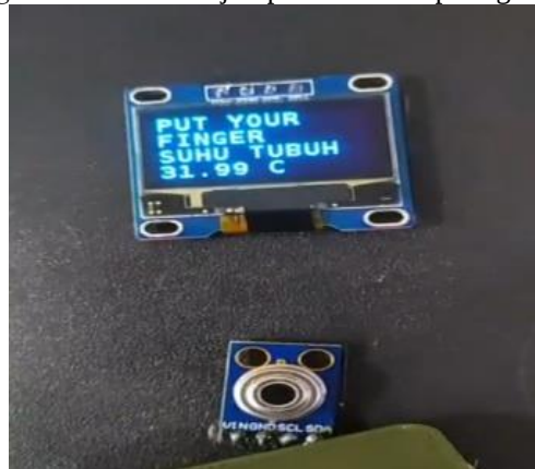
Gambar 7. Tampilan alat siap digunakan
